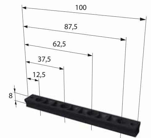
Breite 100 mm, Profil-Nr.: 1.001.004
